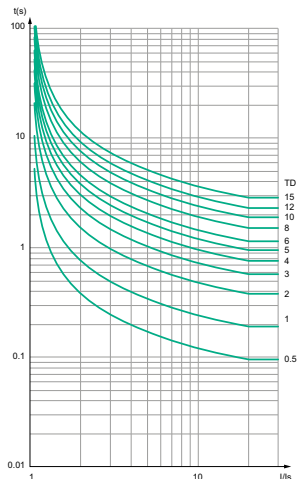
Кривая умеренно обратно-зависимой выдержки времени IEEE (IEEE/MI или МЭК/D)
