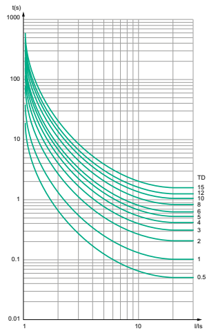
Кривая сильно обратно-зависимой выдержки времени IEEE (IEEE/EI или МЭК/F)
