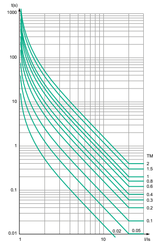
Кривая чрезвычайно обратно-зависимой выдержки времени МЭК (МЭК/EIT или МЭК/C)
