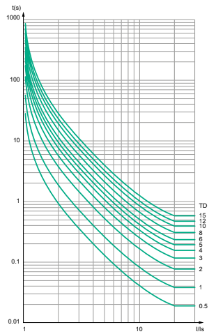
Кривая чрезвычайно обратно-зависимой выдержки времени IEEE (IEEE/VI или МЭК/E)
